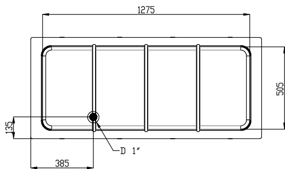
Topp
